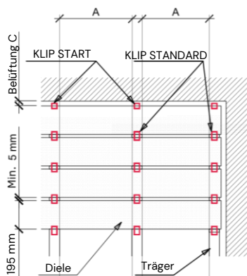
Abb. 4 Mindestabstände zwischen den Dielen sowie zwischen den Dielen und der festen Wand
