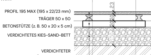
Abb. 1 Aufbau der Terrasse bei Verwendung von Terafest®-Trägern 50x50 mm
